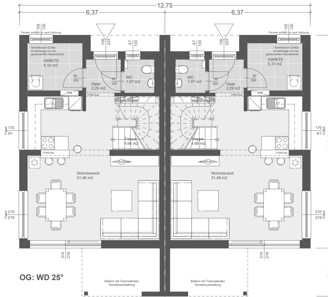
EG - Variante Balkon
